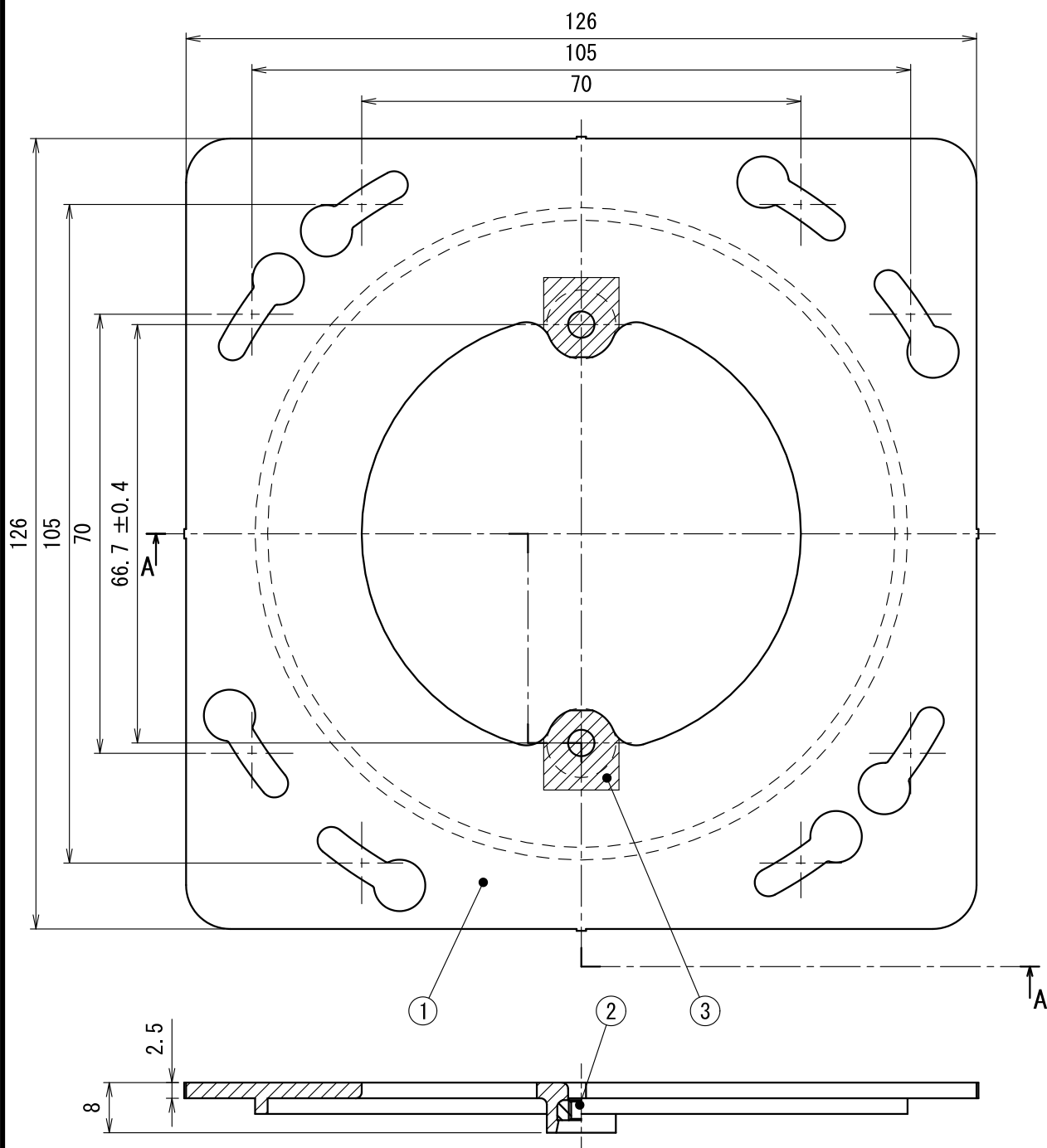
A-A断面図
